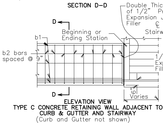
SECTION D-D
